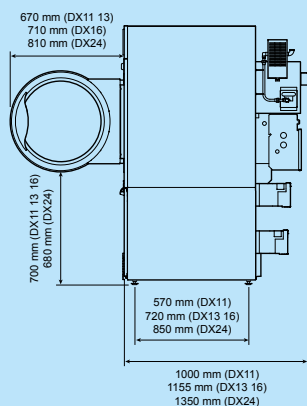
Vedere din lateral DX 11 13 16 24
