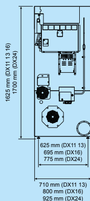
Vedere din spate DX 11 13 16 24
